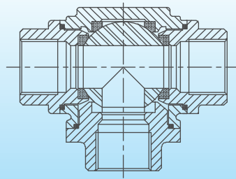
T-port
